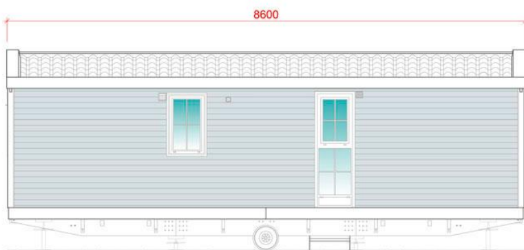
ALZADO TRASERO
