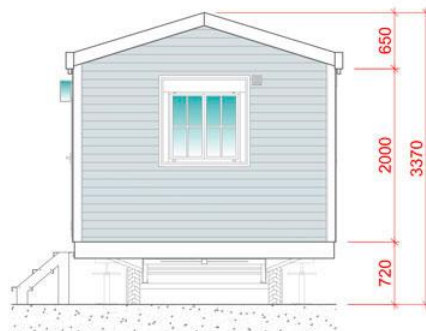
PERFIL DERECHO
