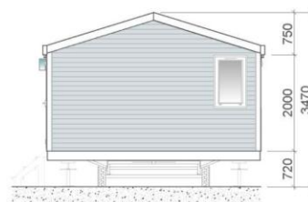
PERFIL DIREITO
